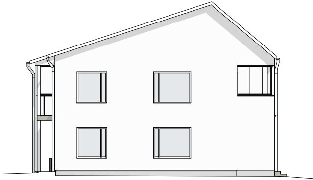
JULKISIVU TALO B LUOTEeseen 1:200
