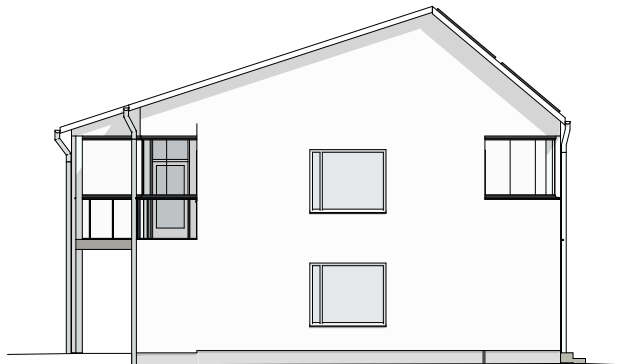
JULKISIVU TALO C LUOTEeseen 1:200
